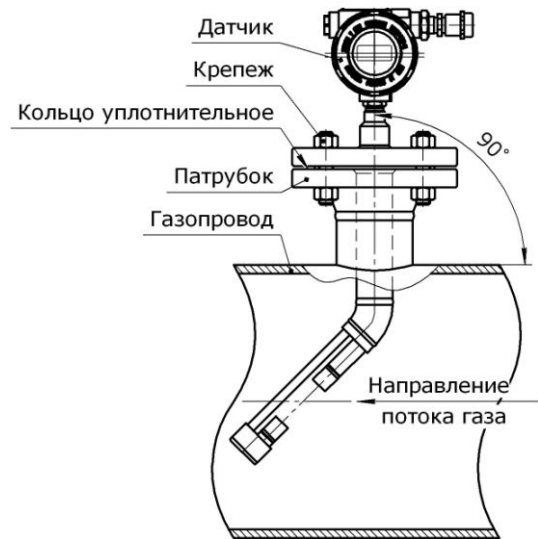
Рисунок 17. Установка датчика исполнения «В»
