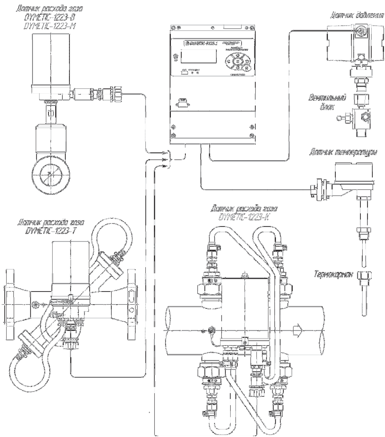
Рисунок 1 Состав счетчика
